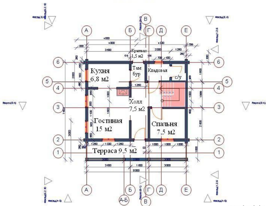
План 1 Этажа
